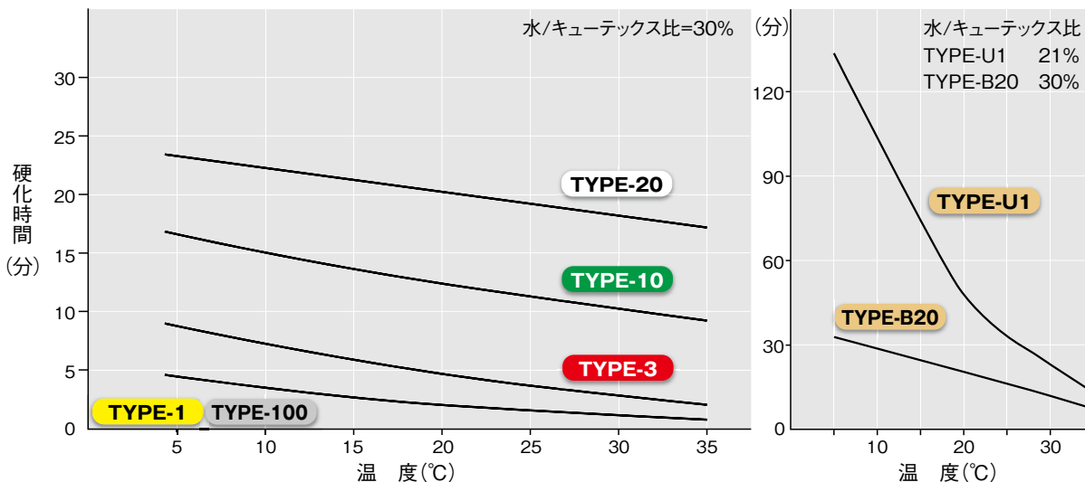
温度と硬化時間の関係
