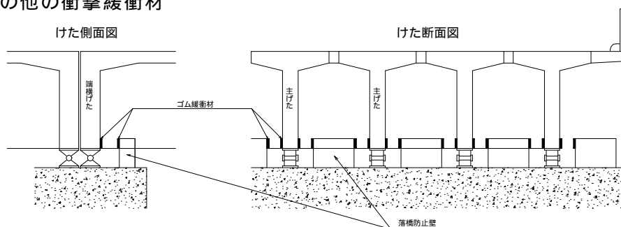
図：落橋防止壁設計例
